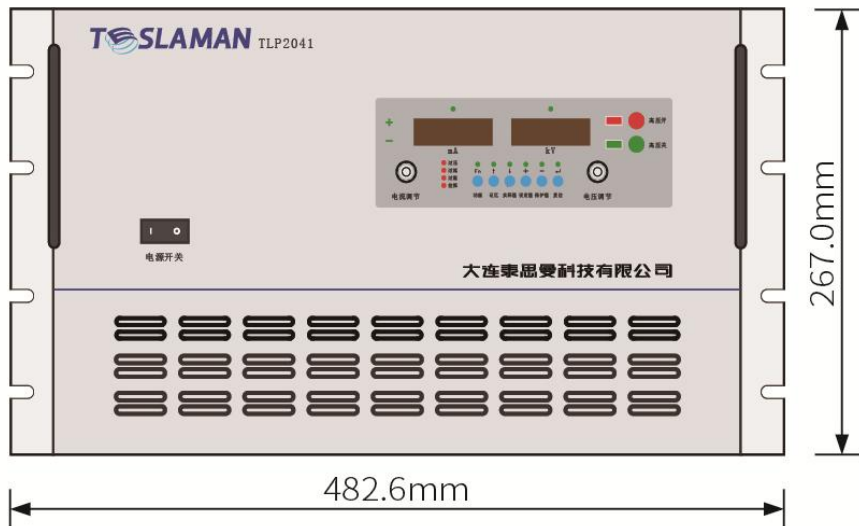
前视图
