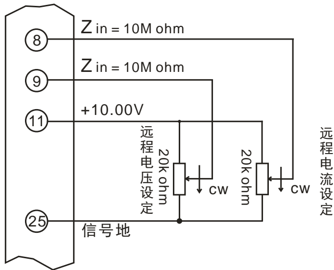
图 6 使用内部电压基准、外部电位器控制
