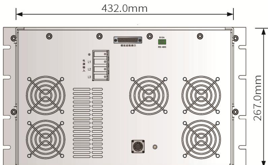
后视图
